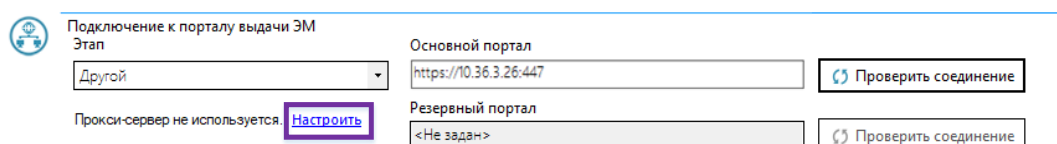
Рис. 3.11 Ссылка «Настроить»
